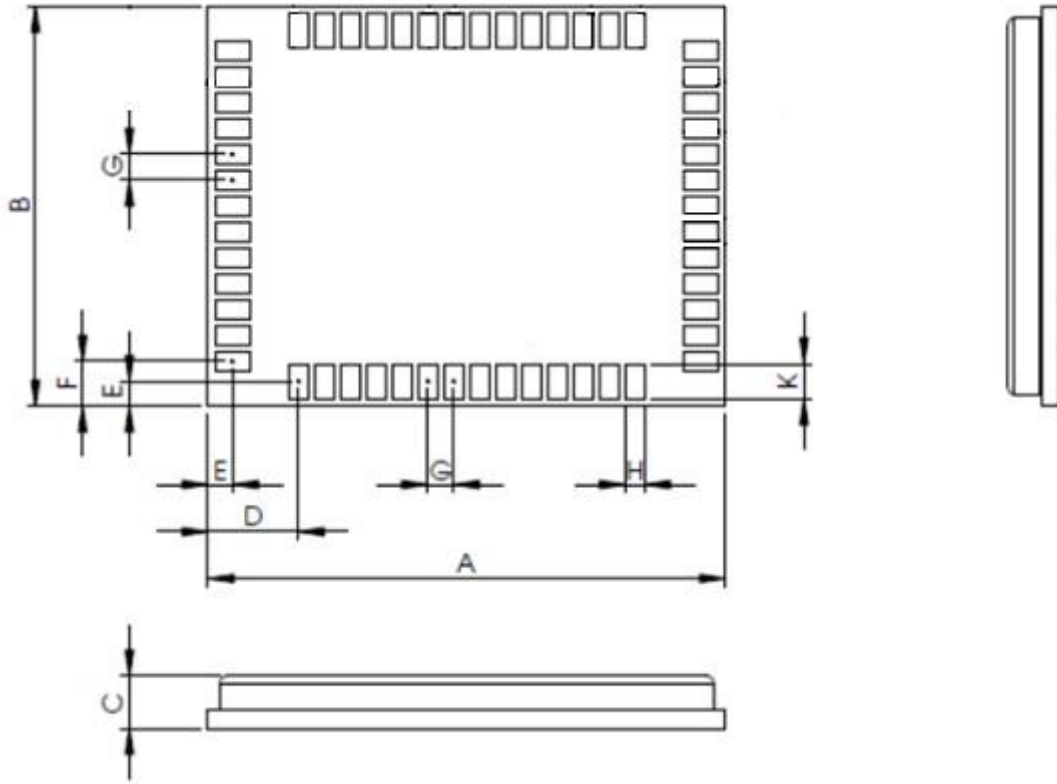
图 6-1 模块外形尺寸及 PCB 封装参考
